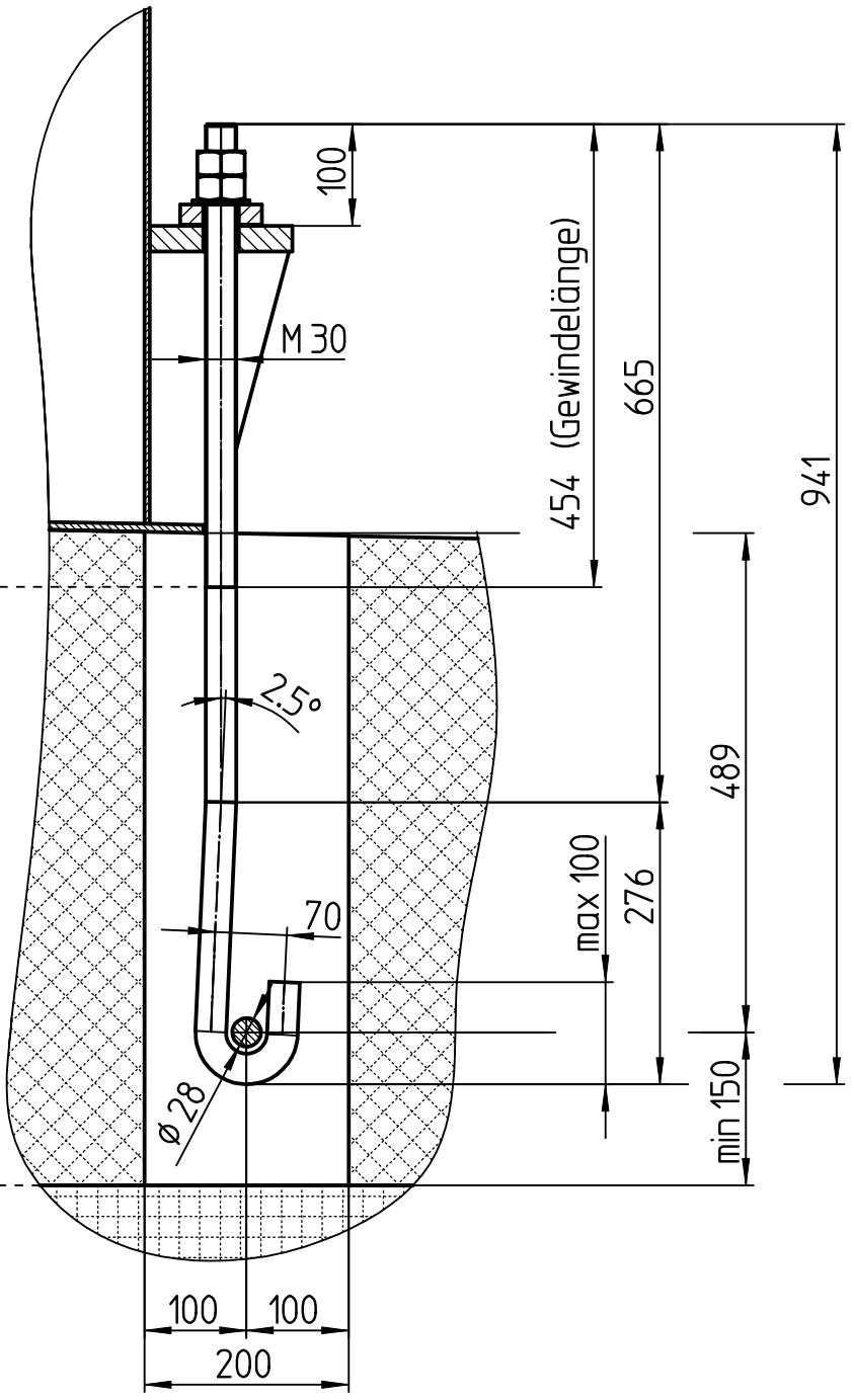
Kürzester Anker M 1:7.5
