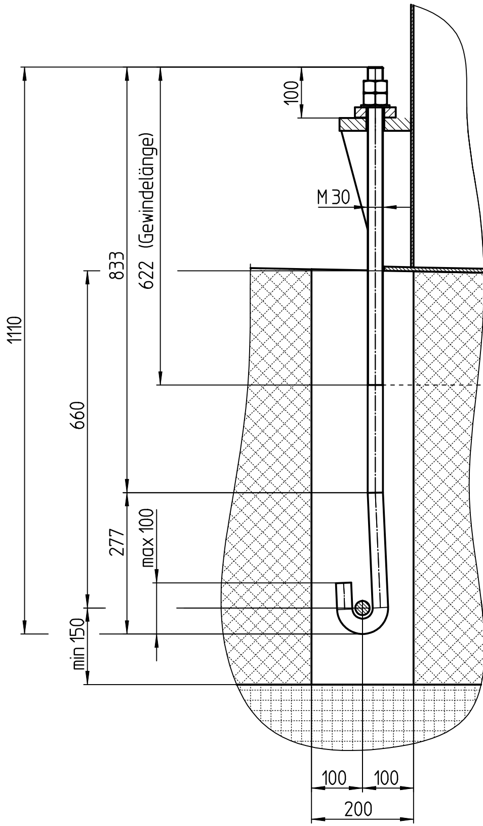
Längster Anker M 1:7.5
